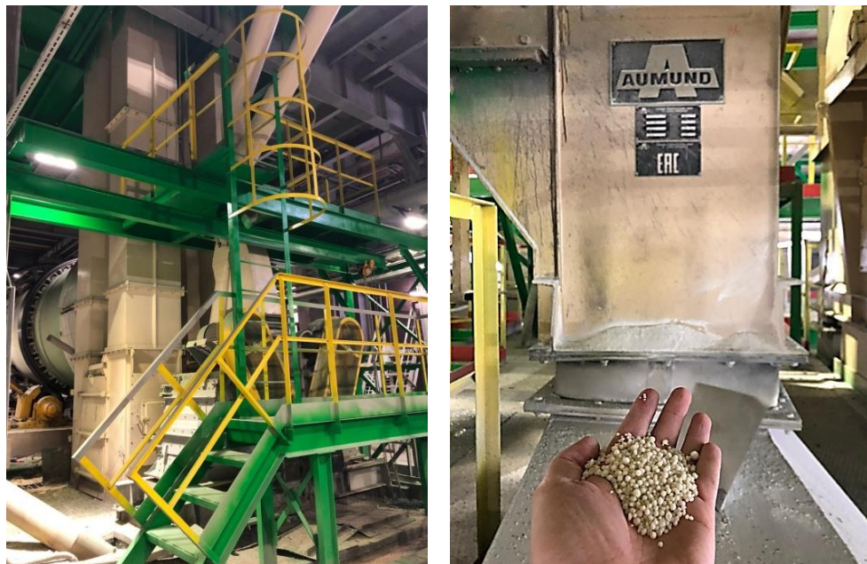
AUMUND-Becherwerke im Einsatz (PhosAgro-Werk Cherepovetz, Foto AUMUND)
